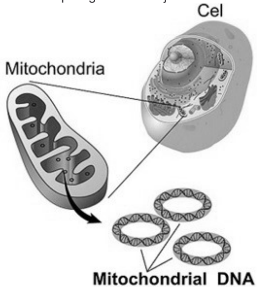
Afb.: Schema van een cel met mitochondriën; de ringen bevatten het mtDNA in de vorm van een dubbele helix. Bron: National Human Genome Research Institute, via Wikimedia Commons.
